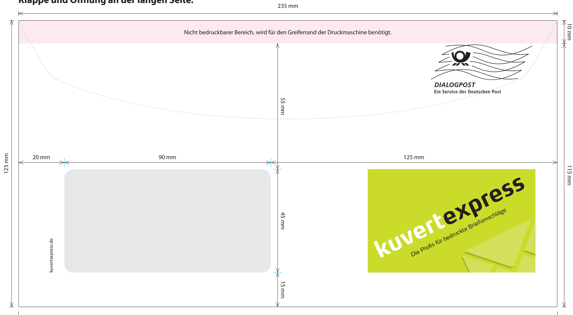
Haftklebung (HK)
